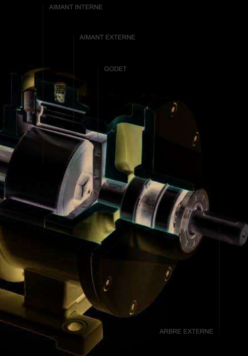
AIMANT INTERNE
